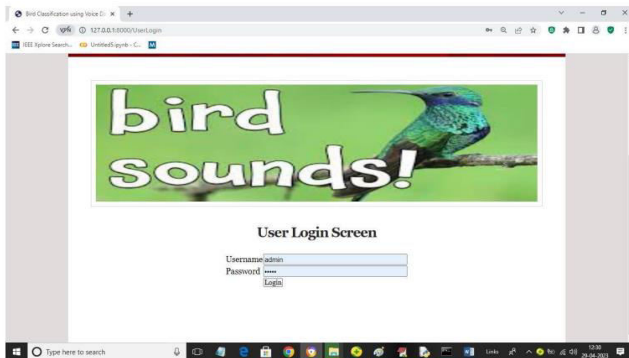
Fig 2. Login page
