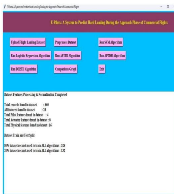
Fig.4. Preprocessing data.
